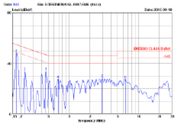
CISPR22 CLASS B AV 230V/50Hz 100% LOAD MARGIN: >6 dB
