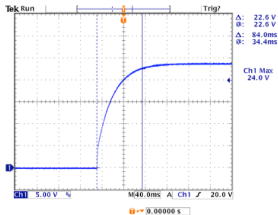
24V Rise Time
