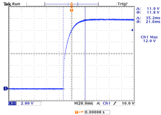
12V Rise Time
