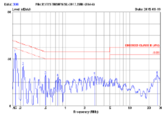
CISPR22 CLASS B AV 230V/50Hz 100% LOAD MARGIN: >9 dB
