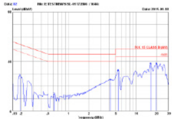
FCC15 CLASS B AV 120V/60Hz 100% LOAD MARGIN: >13 dB
